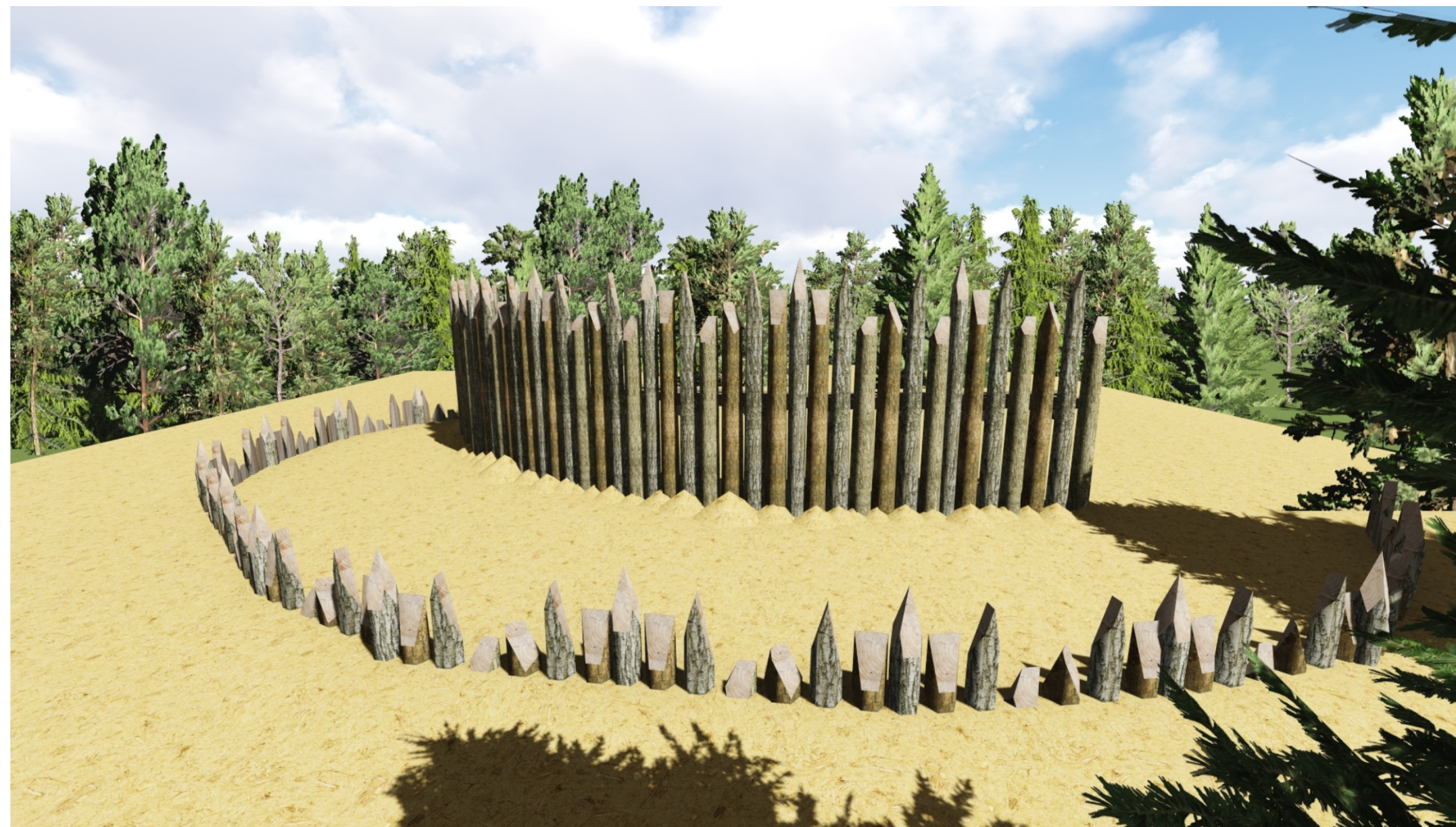
Replika opevnenia hradu „palisáda“ - replika palisády zhotovená z kmeňov stromov v rade, osadené do zeme so štrkovo-kamenným obsypom základu.
