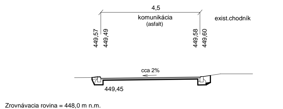
rez 7 (km 0,102)
