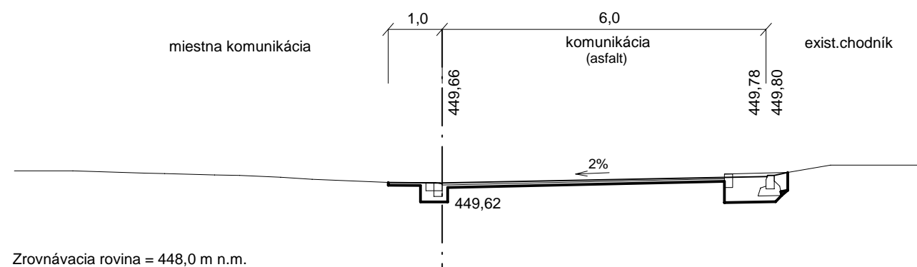
rez 6 (km 0,090)
