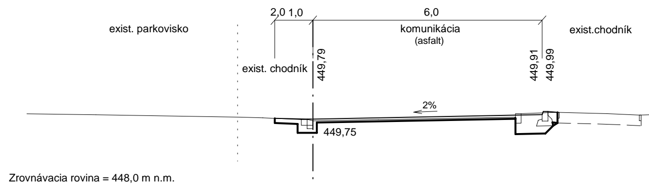
rez 5 (km 0,080)
