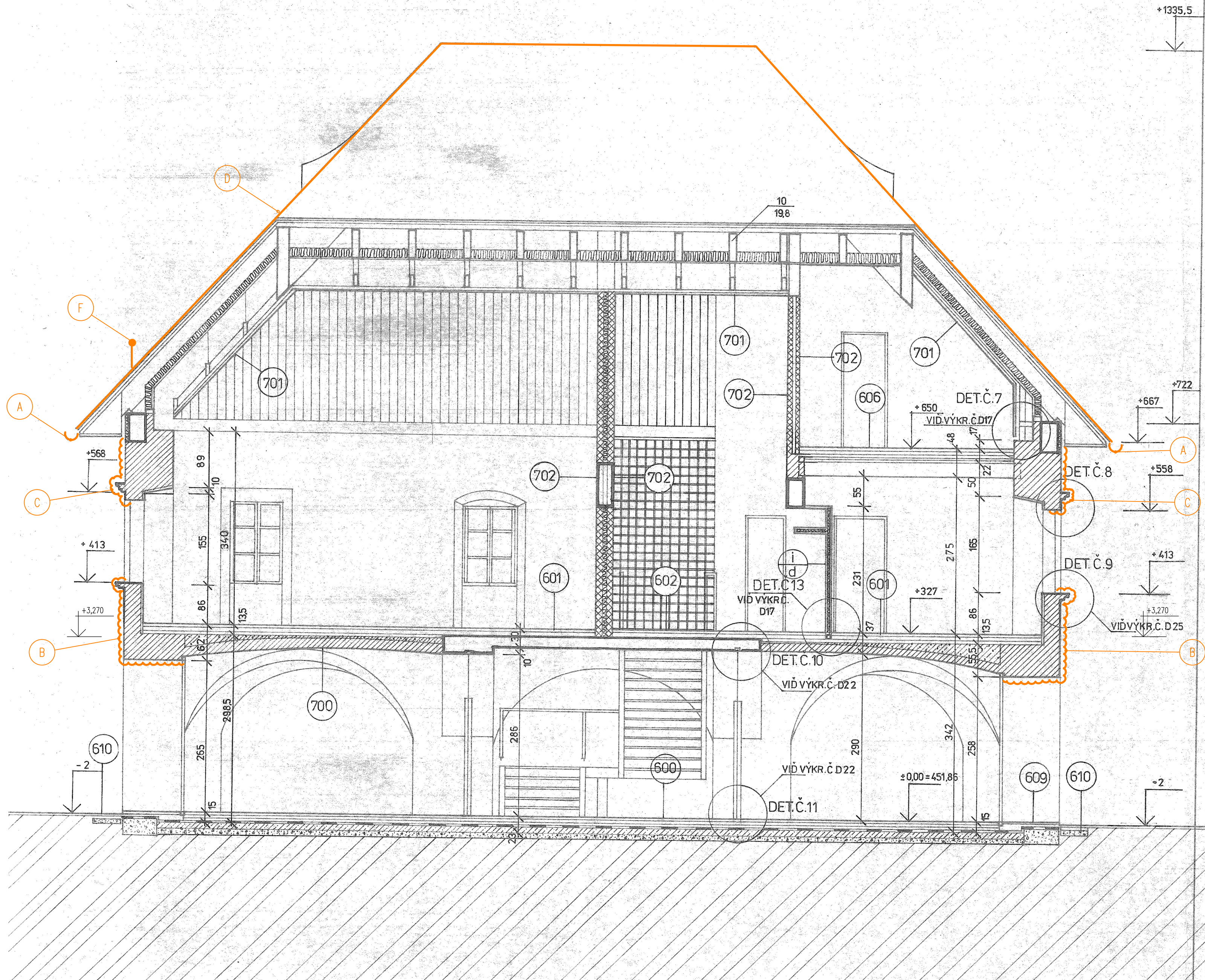
REZ A-A - JESTVUJÚCI STAV A BÚRACIE PRÁCE M 1:50
