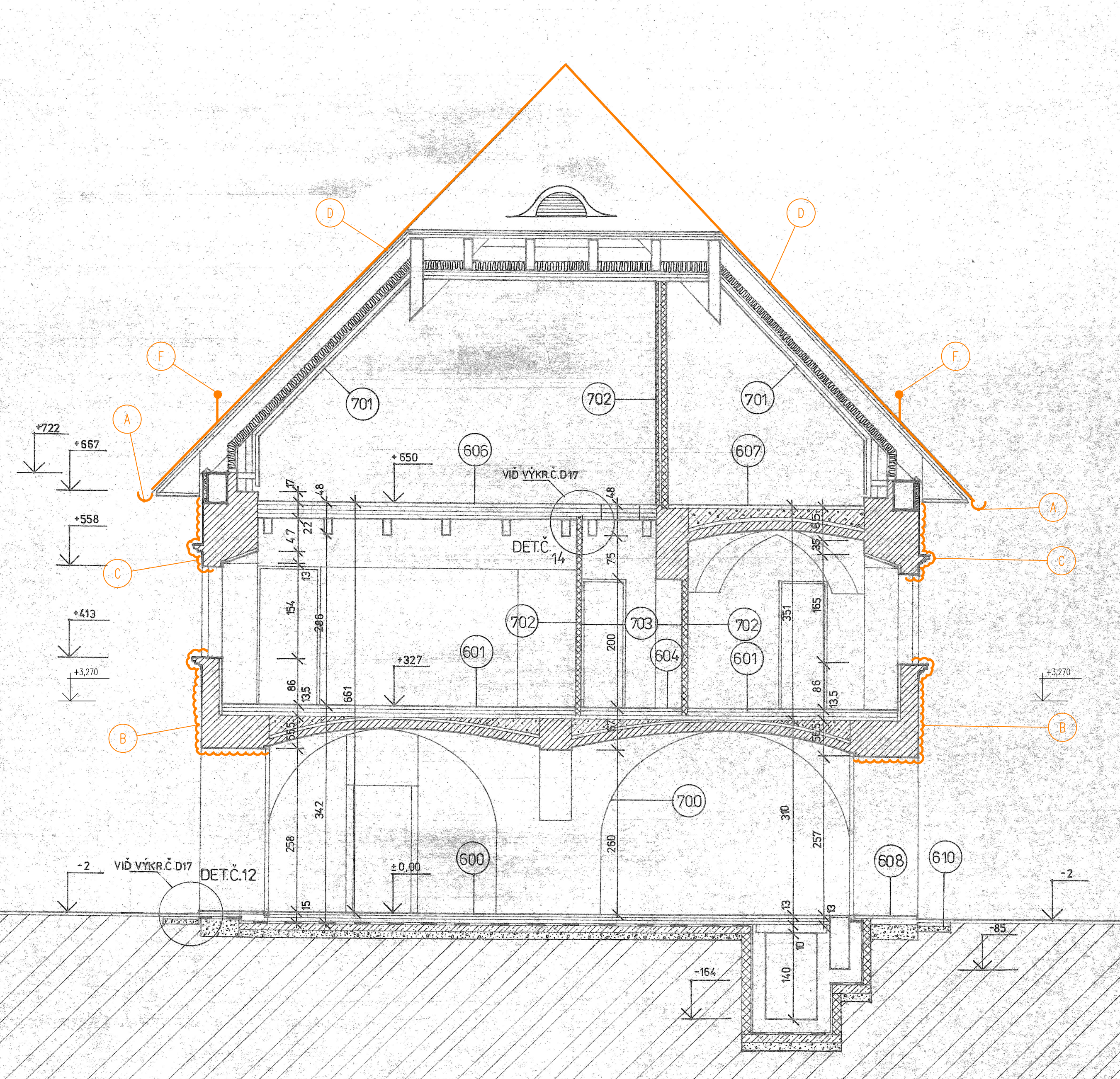
REZ D-D - JESTVUJÚCI STAV A BÚRACIE PRÁCE M 1:50
